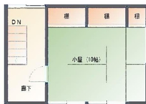
小屋1階
